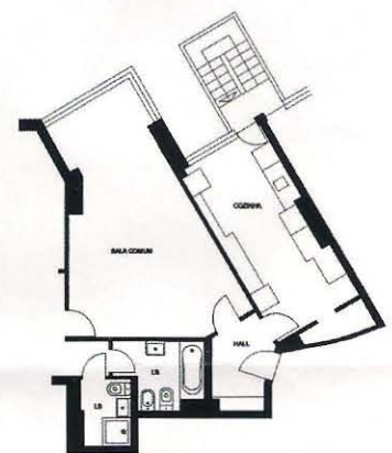
Planta antes das obras
